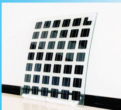
弧形BIPV构件 型号 : DBF(HX)100
